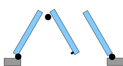
Tre ante a libro, cerniera interna apertura SPINGERE A SINISTRA Spagnoletta di chiusura su ante pieghevoli
