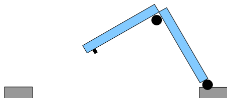
Due ante a libro, cerniera interna apertura SPINGERE A DESTRA
