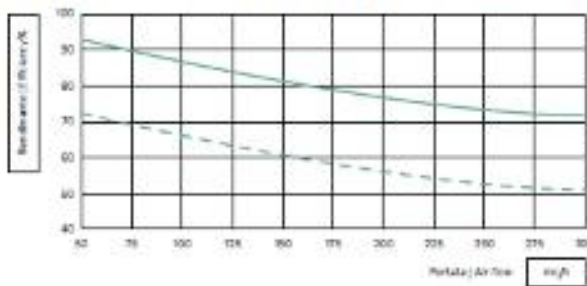
RENDIMENTO INVERNALE DEL RECUPERATORE | WINTER EFFICIENCY OF THE HEAT EXCHANGER
