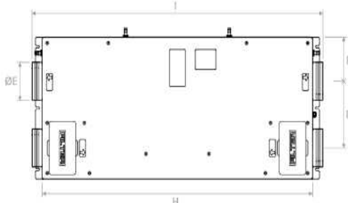
Vista dal basso | Bottom View
