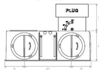
Vista superiore | Top view
