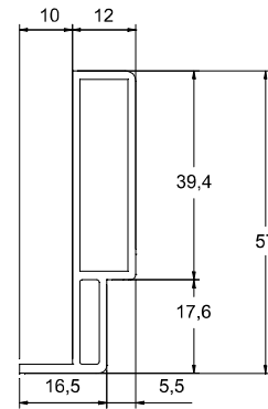
Profilo telaio con battuta 10mm
