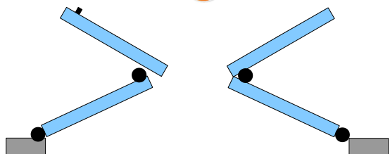
Quattro ante a libro, cerniera esterna apertura SPINGERE A SINISTRA Spagnoletta di chiusura su prima anta ripieghevole SX
