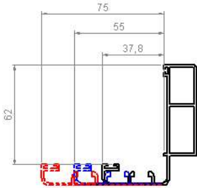
Profilo telaio con battuta 37,8/55/75 mm
