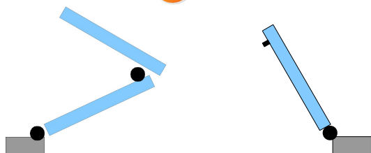
Tre ante a libro, cerniera esterna apertura SPINGERE A DESTRA Spagnoletta di chiusura su anta battente
