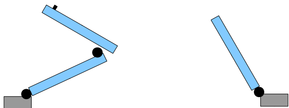
Tre ante a libro, cerniera esterna apertura SPINGERE A SINISTRA Spagnoletta di chiusura su anta pieghevoli
